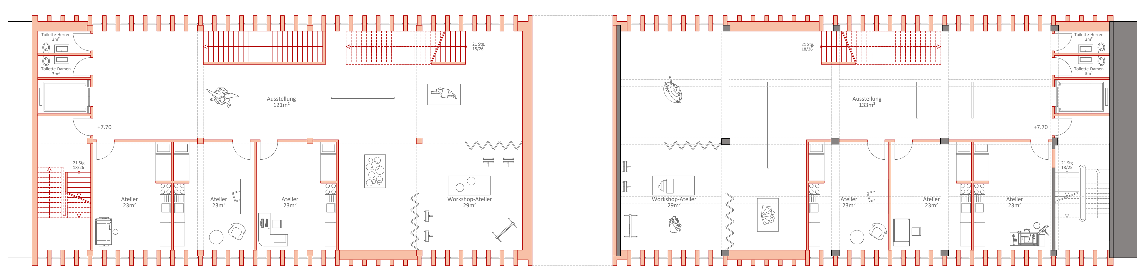
Grundriss 1:100 2. Obergeschoss
