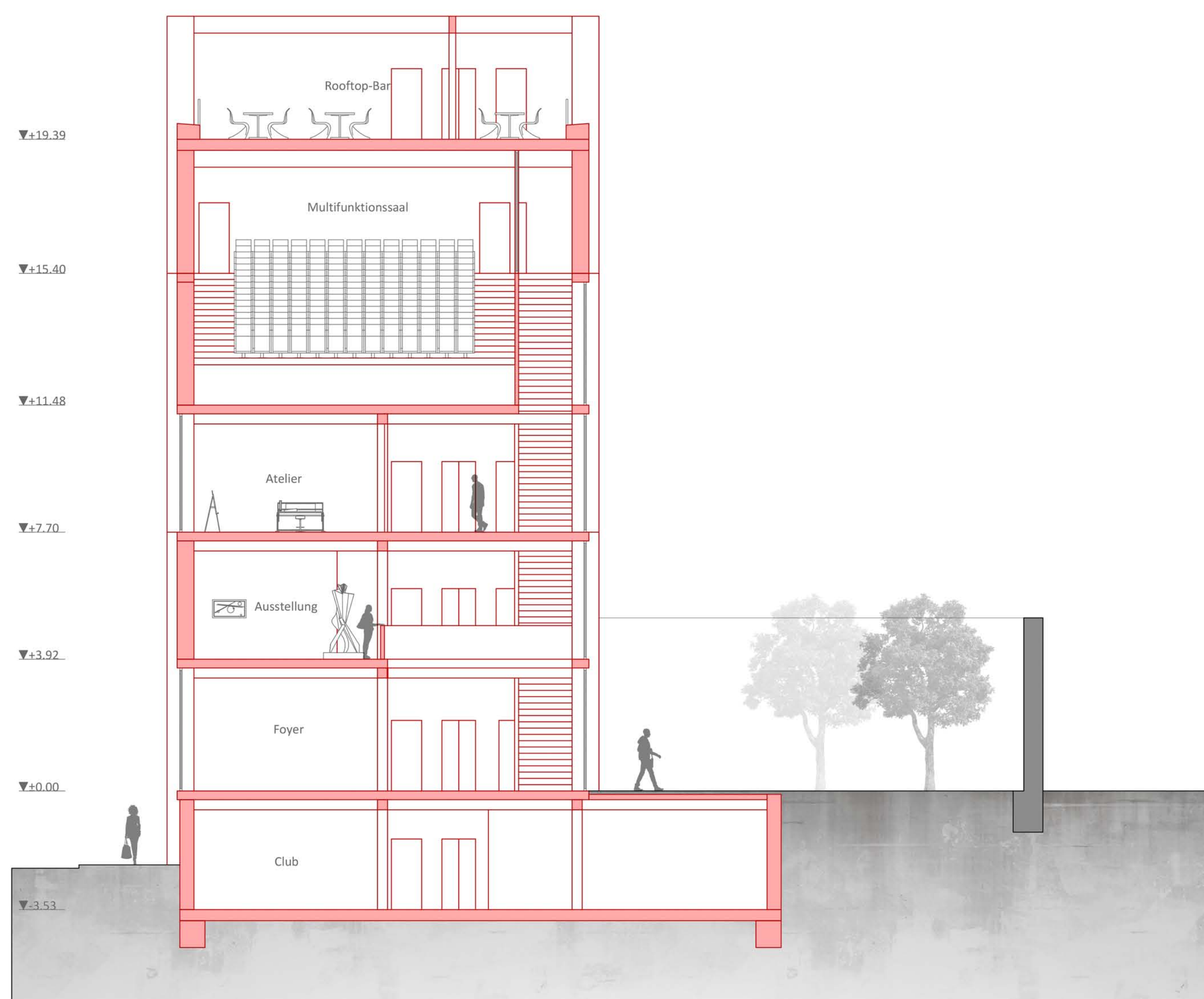
Schnitt b-b 1:100
