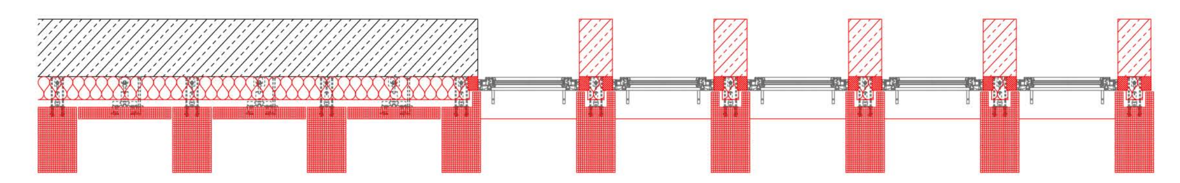
Fassadenschnitt 1:20
