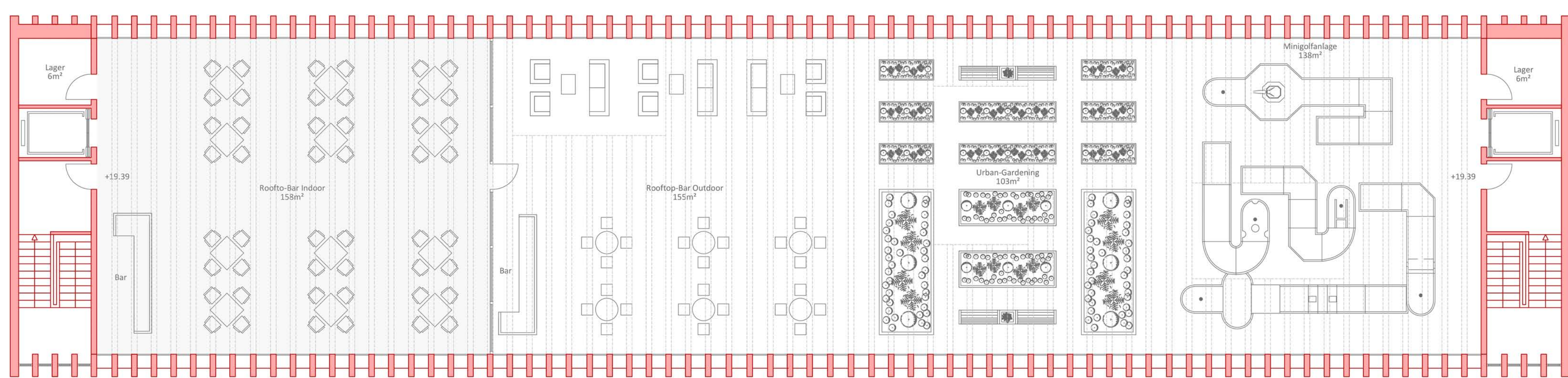
Grundriss 1:100 Dachgeschoss
