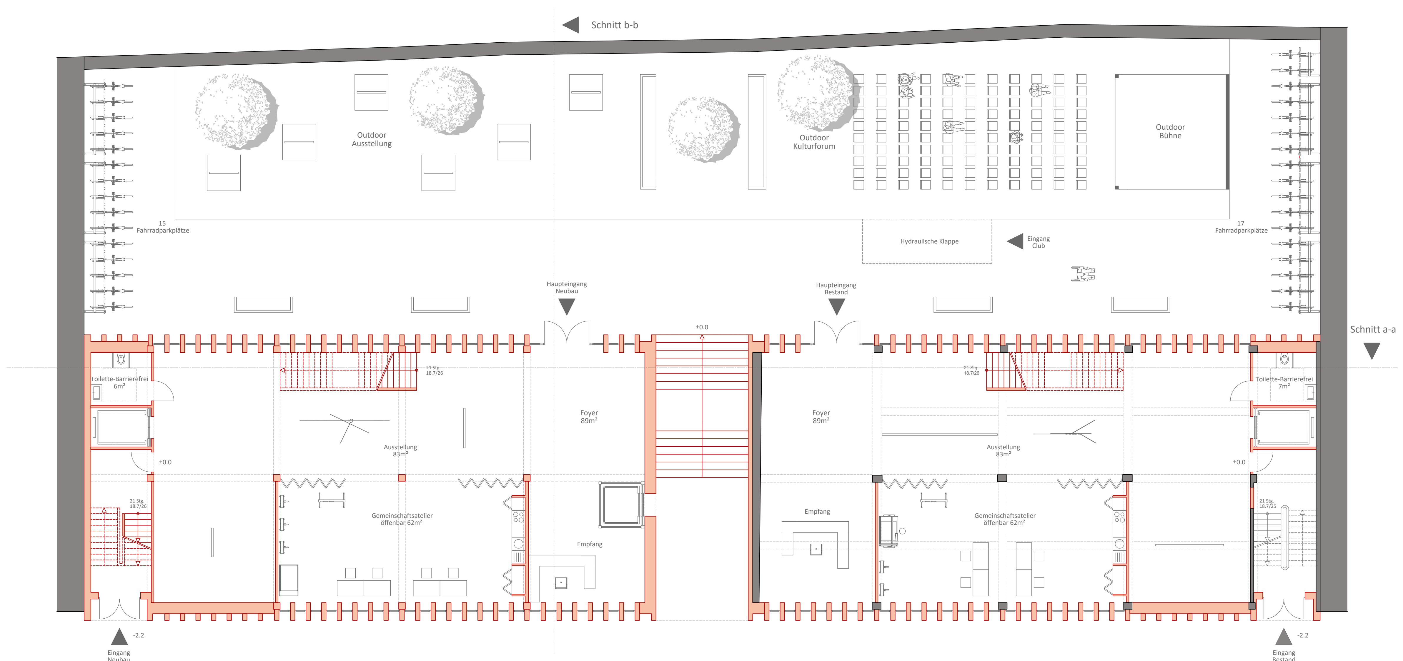
Grundriss 1:100 Erdgeschoss
