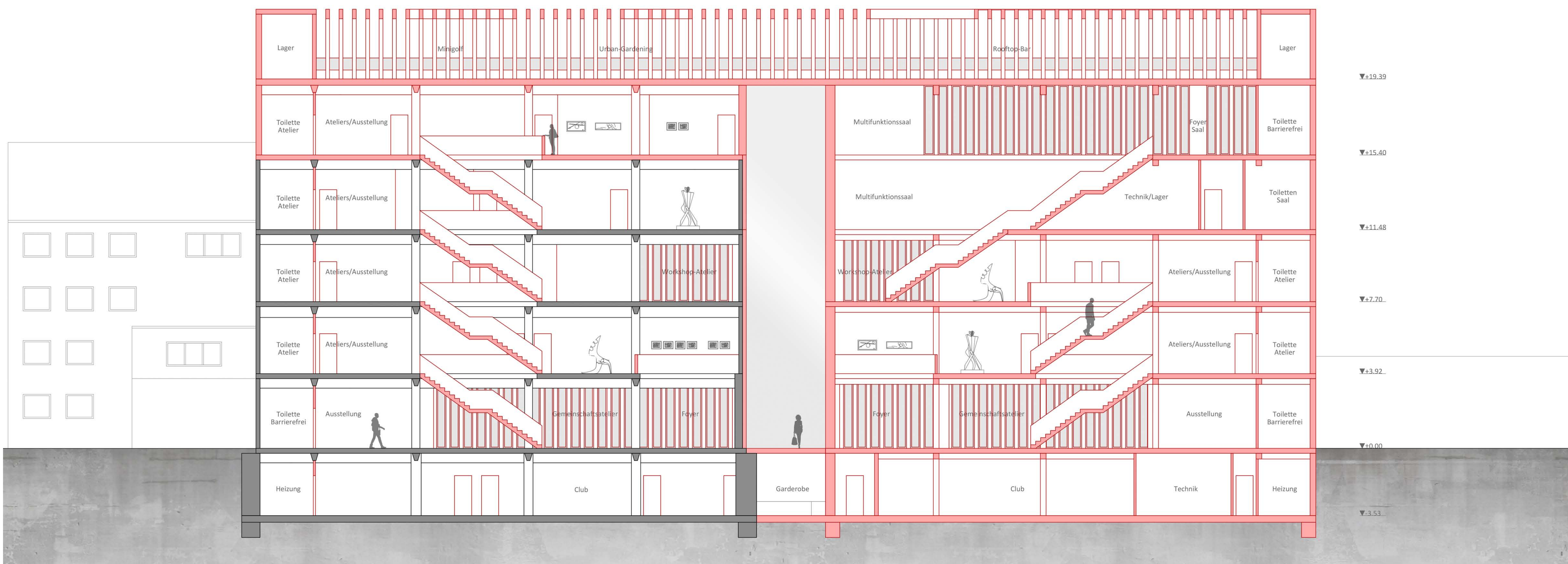
Schnitt a-a 1:100
