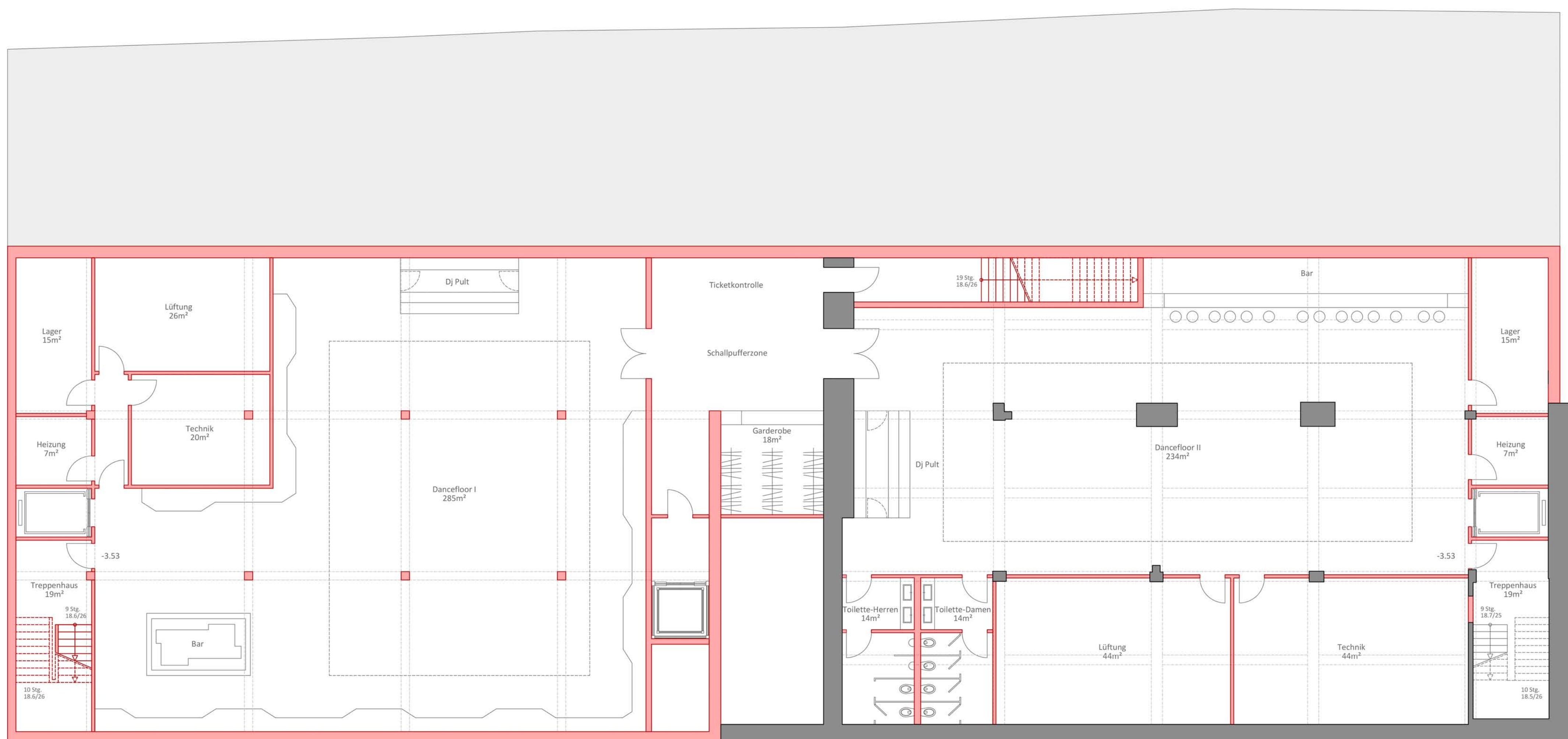
Grundriss 1:100 Untergeschoss
